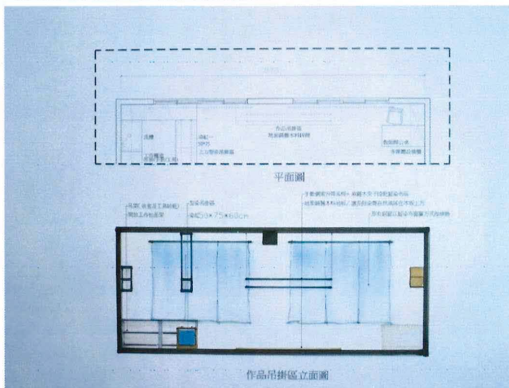
附圖七：藍染教室作品吊掛區細部設計規劃圖
