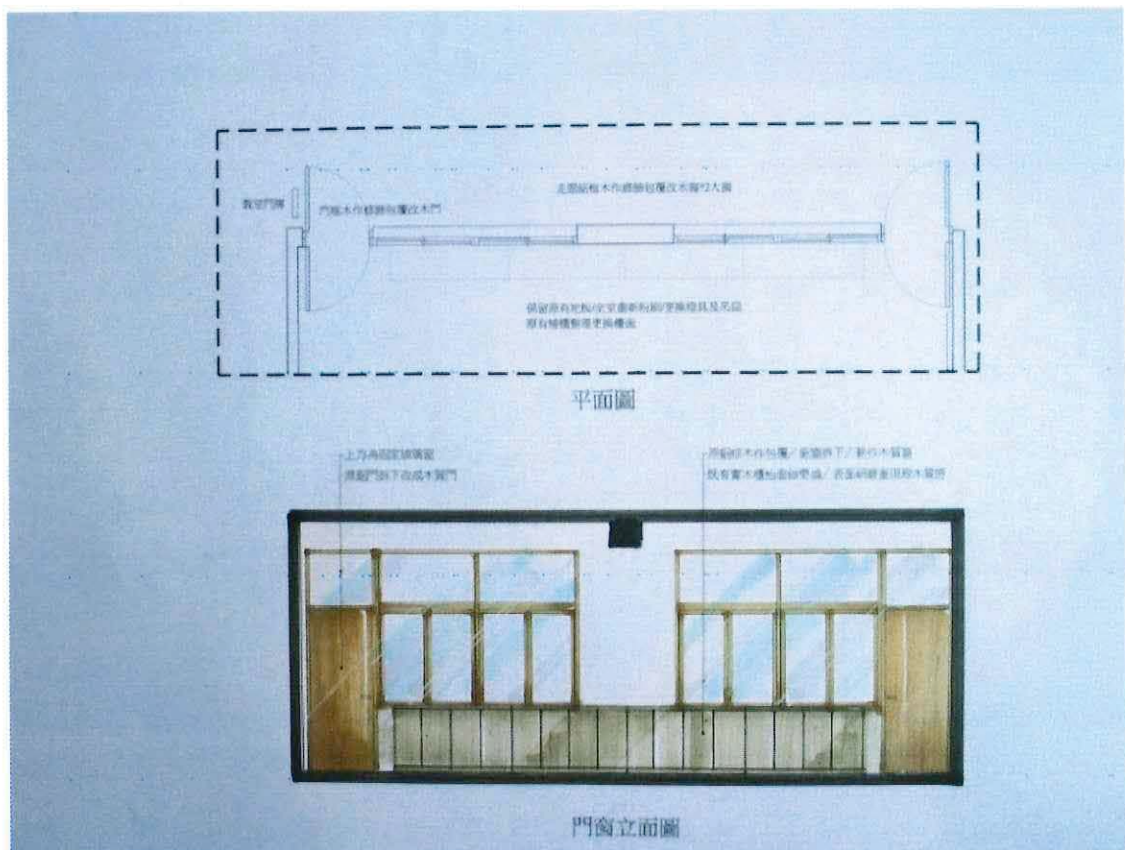
附圖六：藍染教室工作收納區細部設計規劃圖
